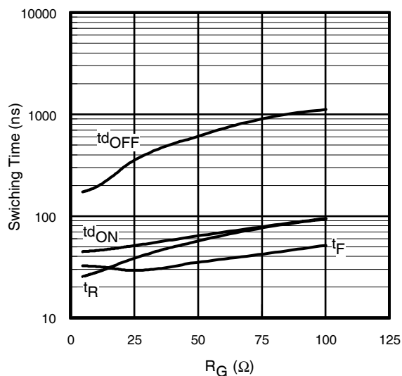
Fig. 15 - Typ. Switching Time vs. R_G T_J = 150^\circ\text{C} ; L=200\mu\text{H} ; V_{CE}=400\text{V} I_{CE}=30\text{A} ; V_{GE}=15\text{V}
