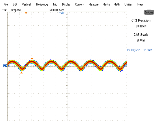
Fig. 20. Output Voltage Ripple, 2A load Ch 2 : V_o
