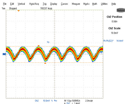
Fig. 20. Output Voltage Ripple, 3A load Ch2: V_o
