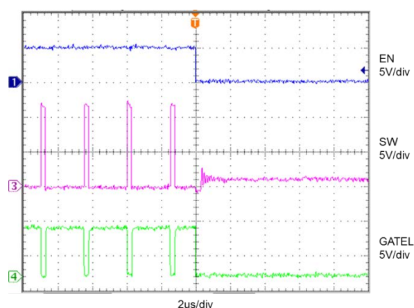
Figure 29: Enable (EN) Delay, 0A
