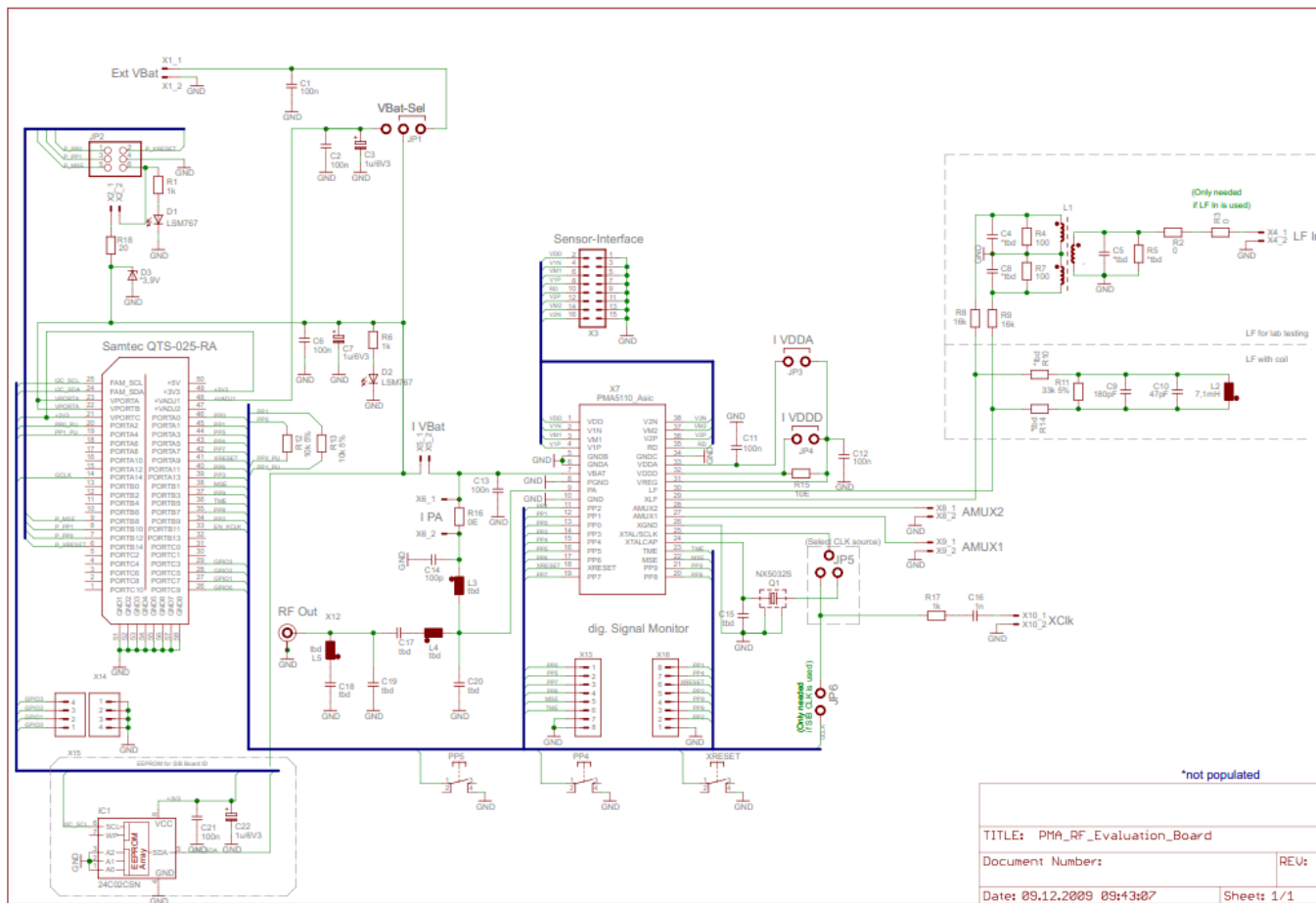
图6 PMA 射频评估板示意图
