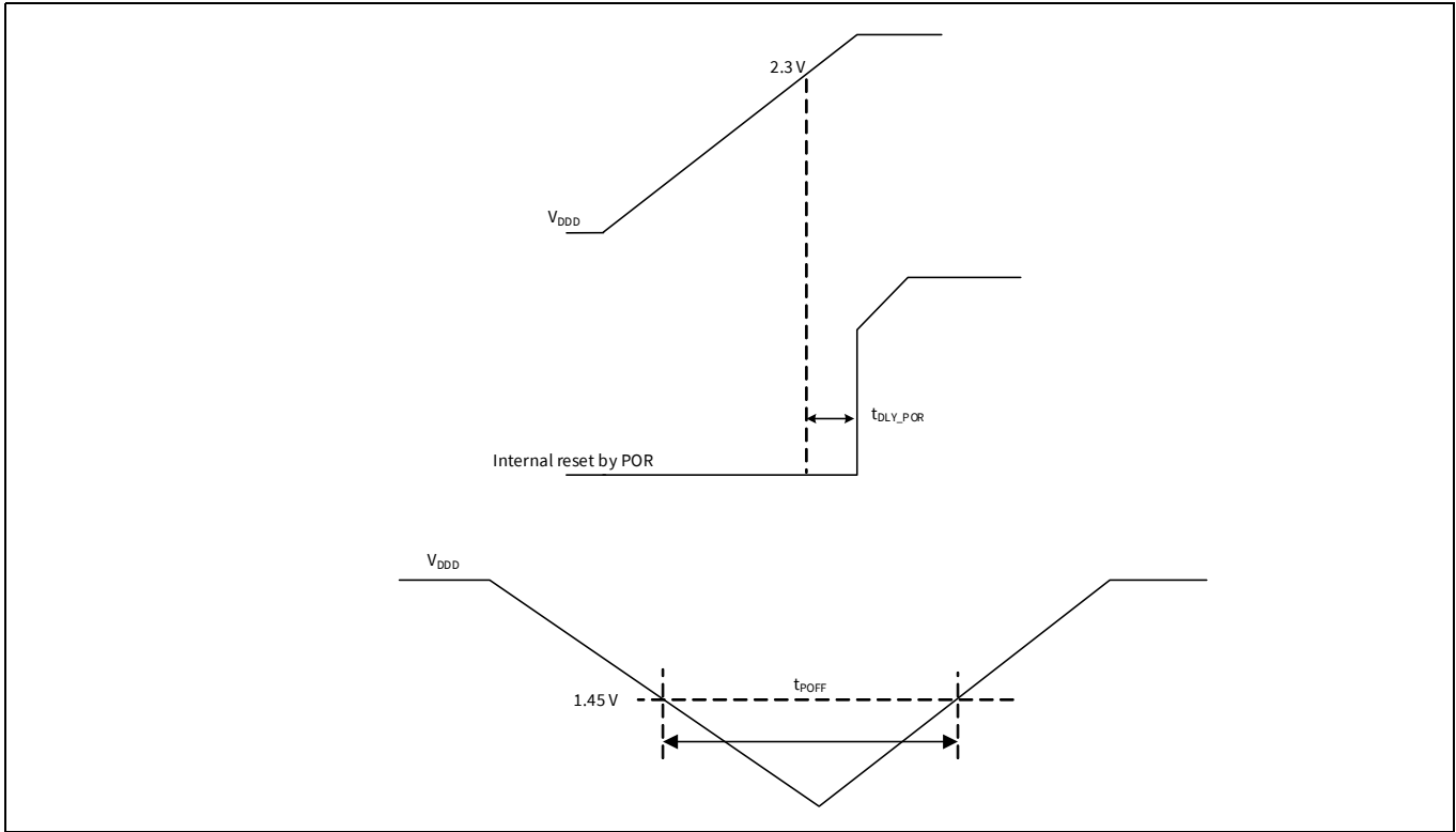
Figure 24 POR specifications
