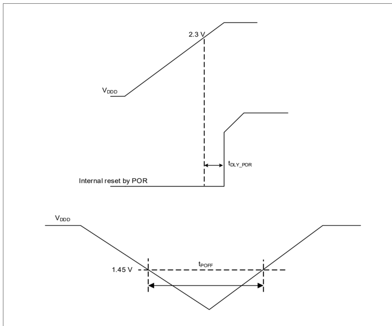
Figure 26 POR specifications
