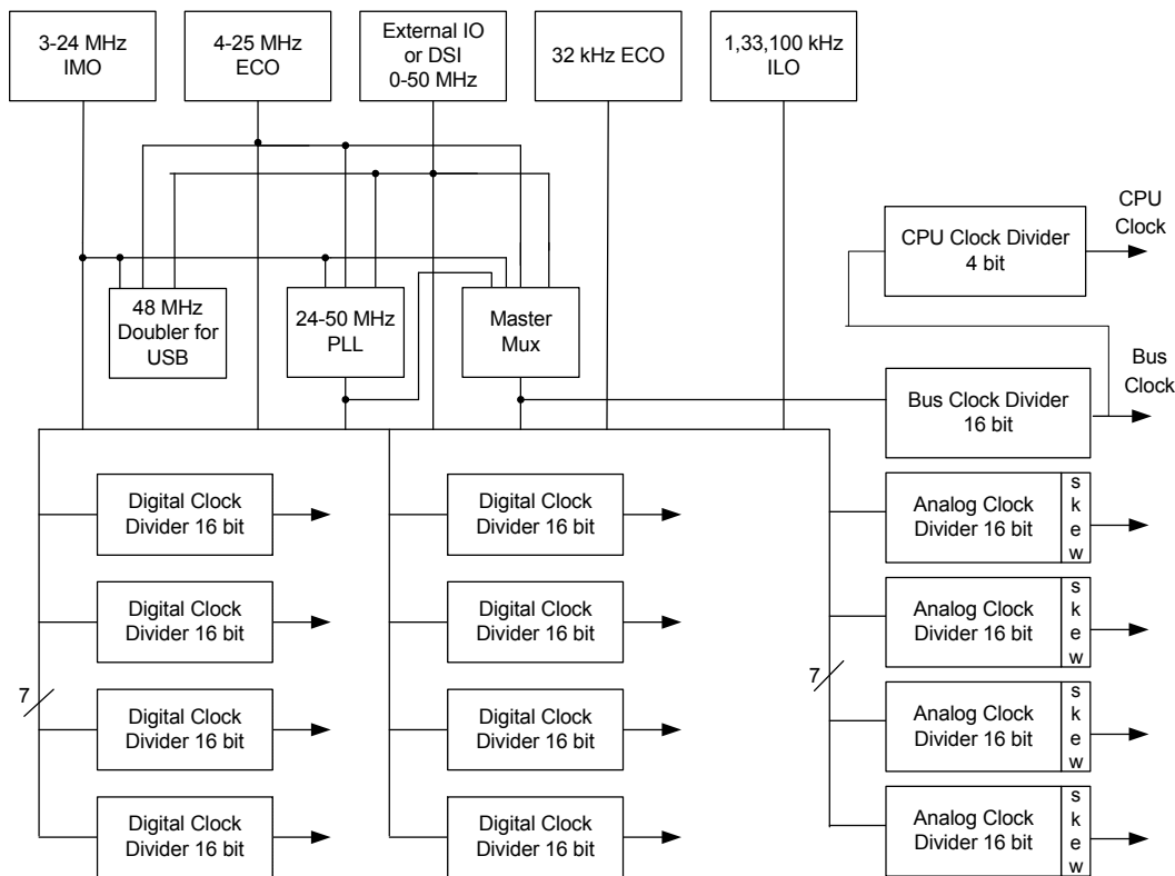
图 6-1. 时钟子系统
