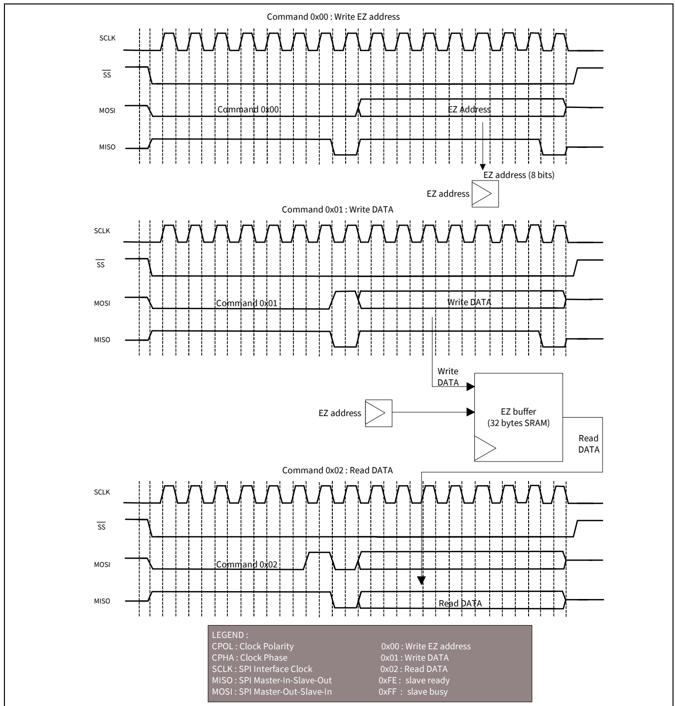
Figure 27-9. EZSPI example
