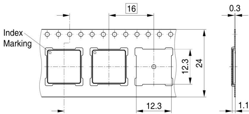
PG-VQFN-70-1, -2-TP V02
