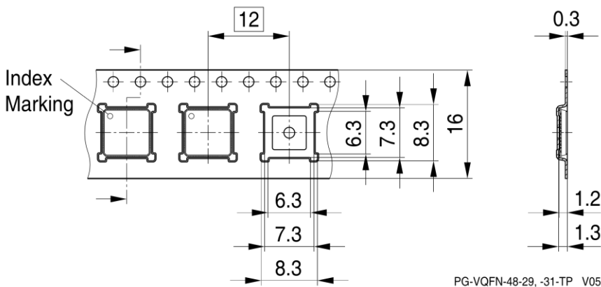
PG-VQFN-48-29, -31-TP V05
