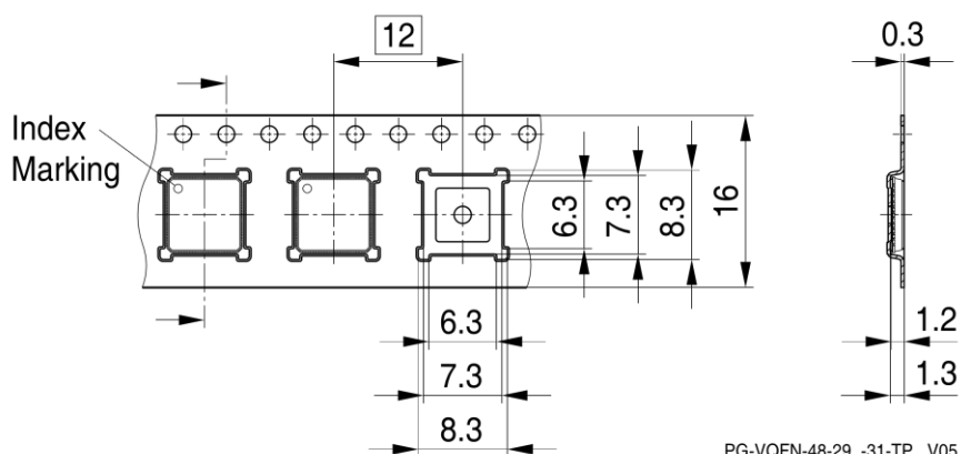
PG-VQFN-48-29, -31-TP V05
