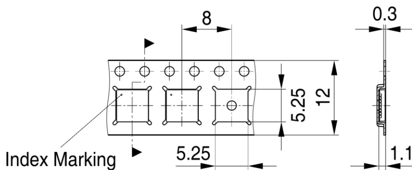
PG-VQFN-32-13-TP V01
