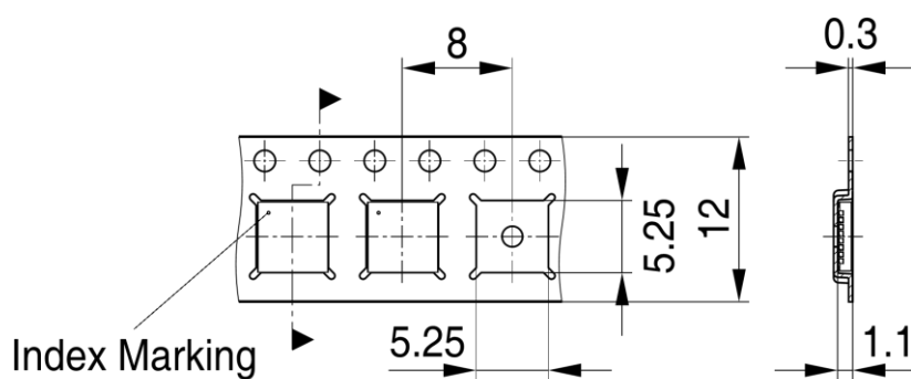
PG-VQFN-32-13-TP V01
