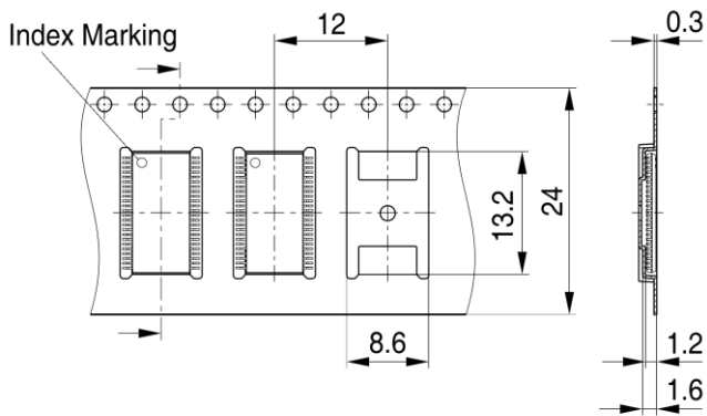
PG-TSSOP-48-2-TP V01
