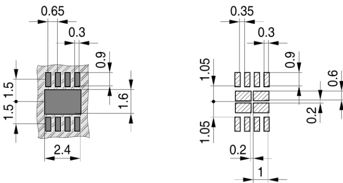
PG-TSON-8-1-FP V01
