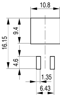
PG-TO263-3-2-FP V03
