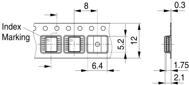
PG-SSOP-14-1,-2,-3,-5-TP V01
