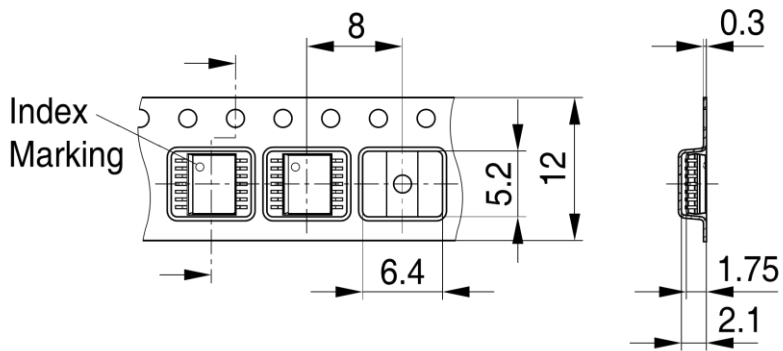
PG-SSOP-14-1,-2,-3,-5-TP V01
