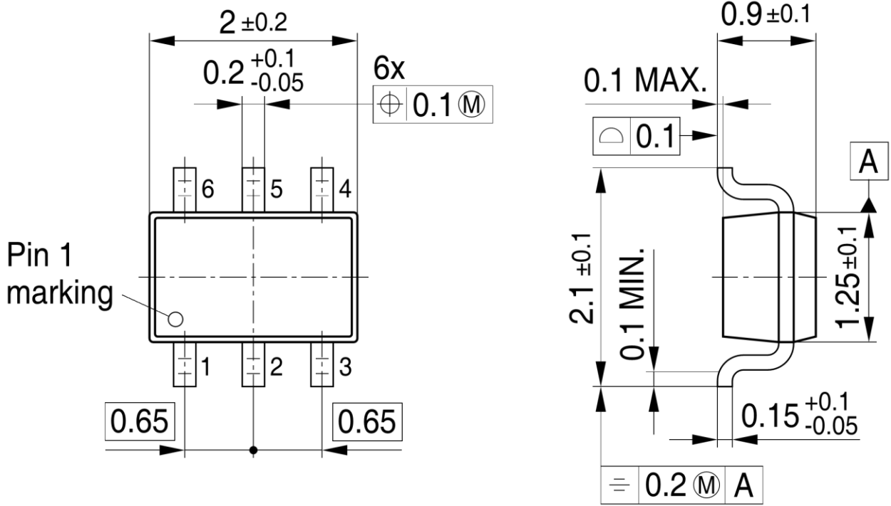
SOT363-PO V06
