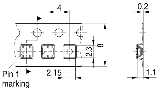
SOT363-TP V02
