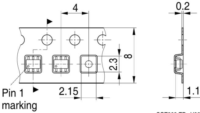
SOT363-TP V02
