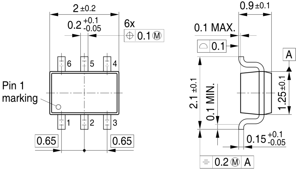
SOT363-PO V06
