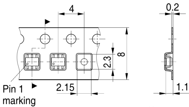
SOT363-TP V02
