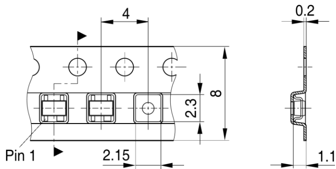
SOT323-TP V02
