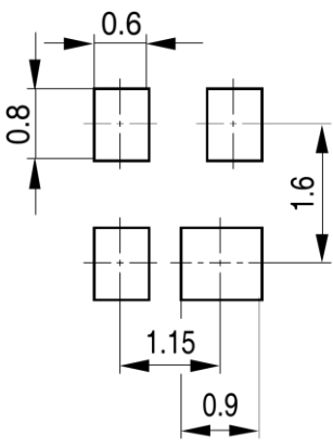
SOT343-FP V08
