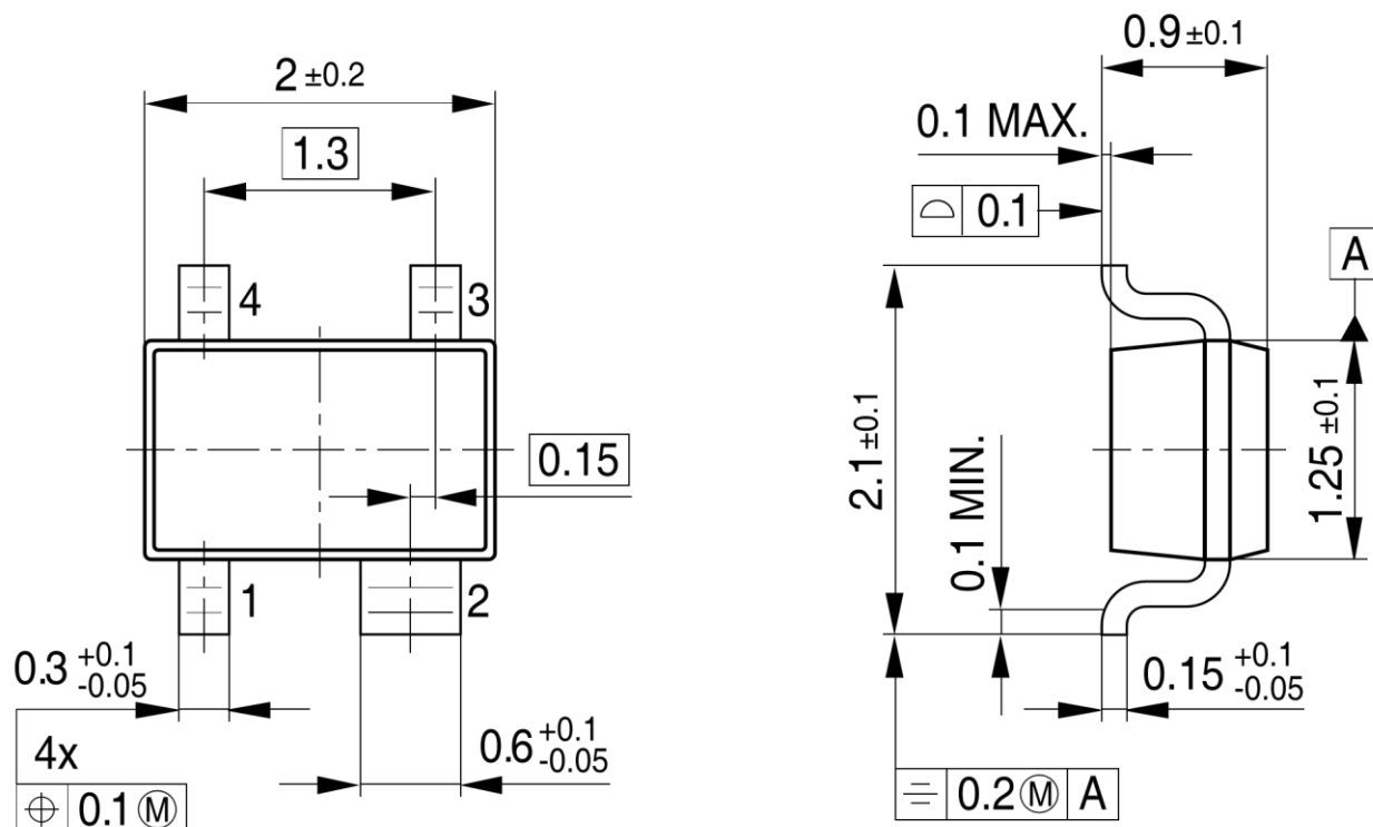
SOT343-PO V08
