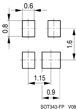
SOT343-FP V08
