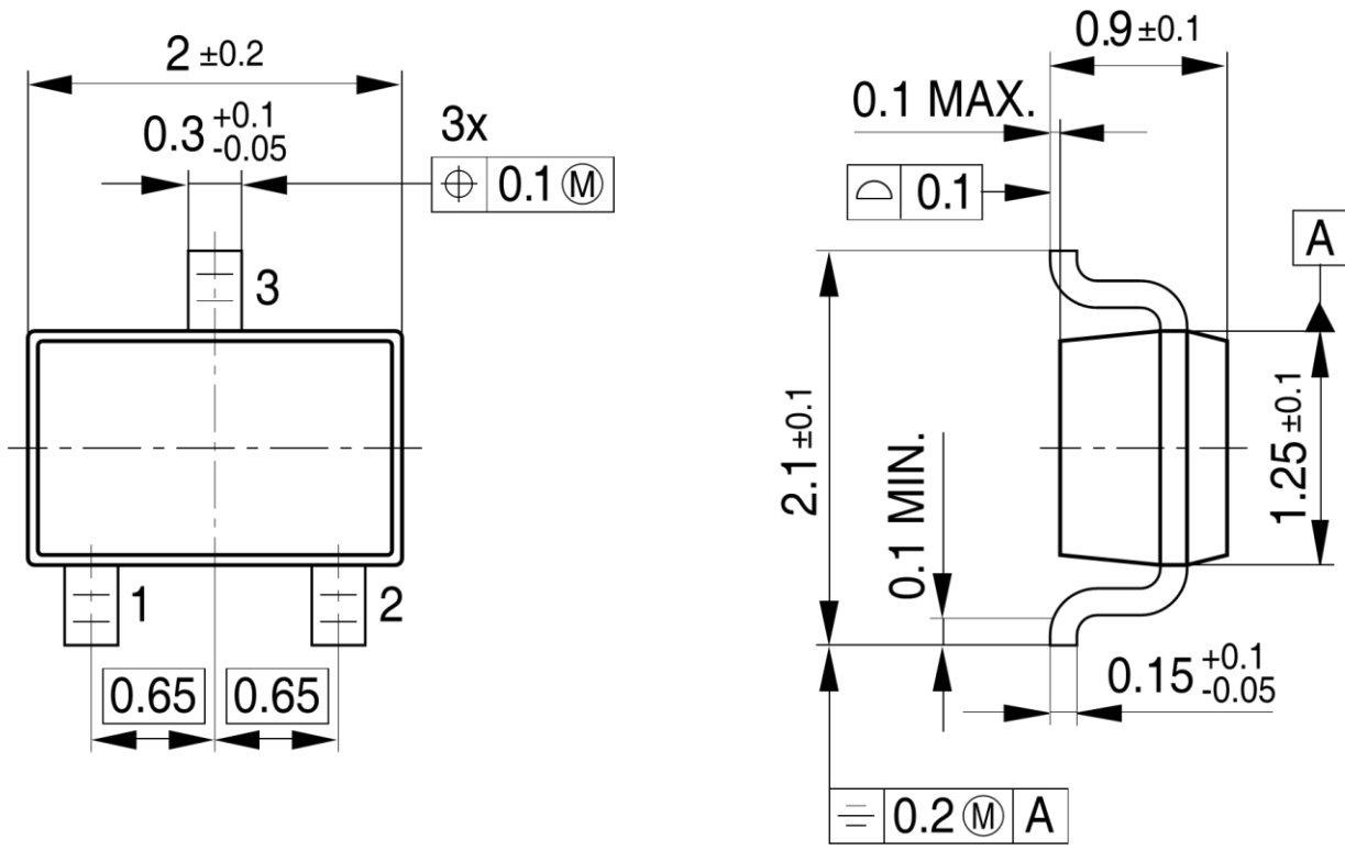
SOT323-PO V08
