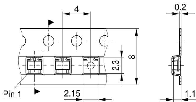
SOT323-TP V02
