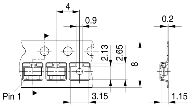
SOT23-TP V02
