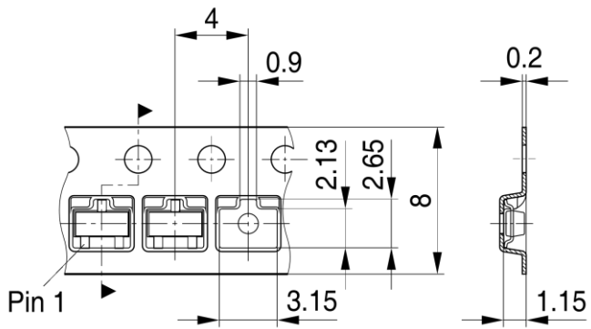
SOT23-TP V02
