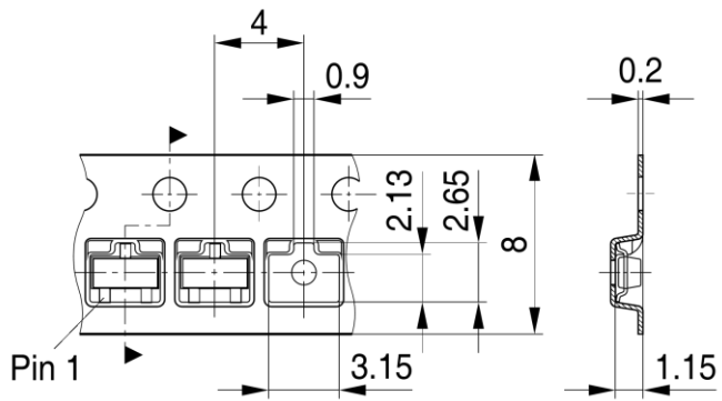
SOT23-TP V02
