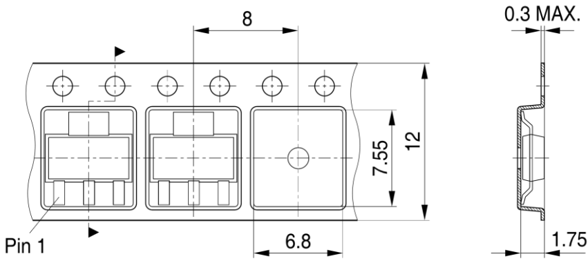
SOT223-TP V03
