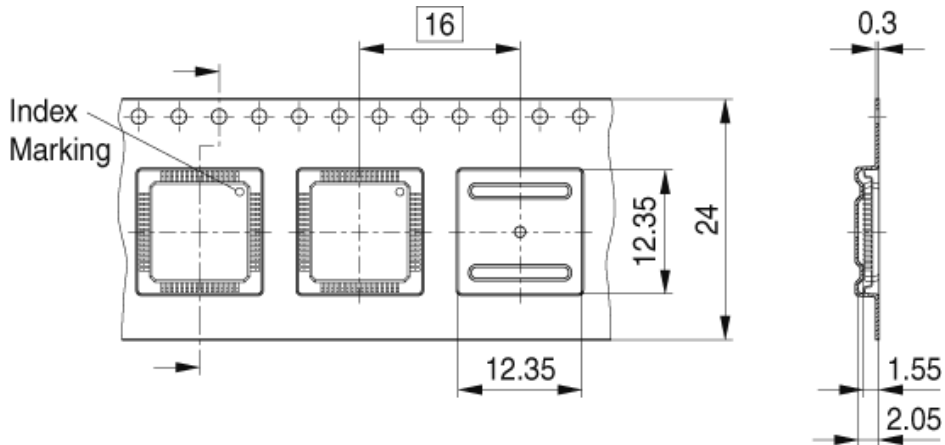
PG-LQFP-64-10, -21, -26-TP V05
