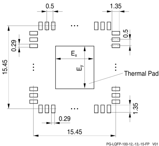
PG-LQFP-100-12,-13,-15-FP V01
