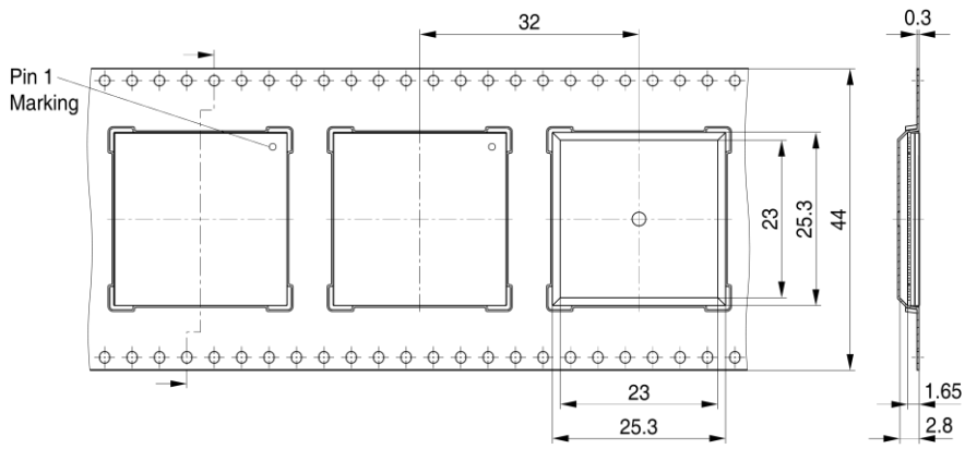
PG-LFBGA-516-1, -2, -3, -4, -5-TP V01
