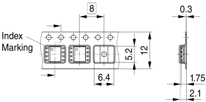
PG-DSO-8-41, -42, -51, -53, -58-TP V09
