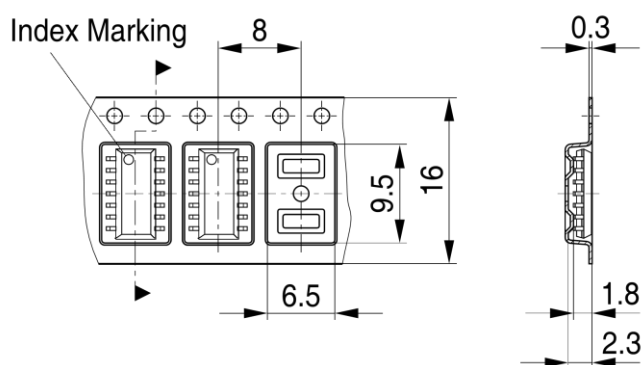
PG-DSO-14-1, -22, -30, -31, -32, -35, -36, -37-TP V05
