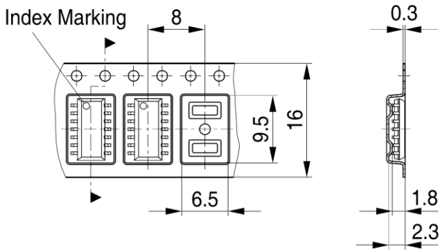
PG-DSO-14-3, -8, -9, -11, -14, -23, -24-TP V05
