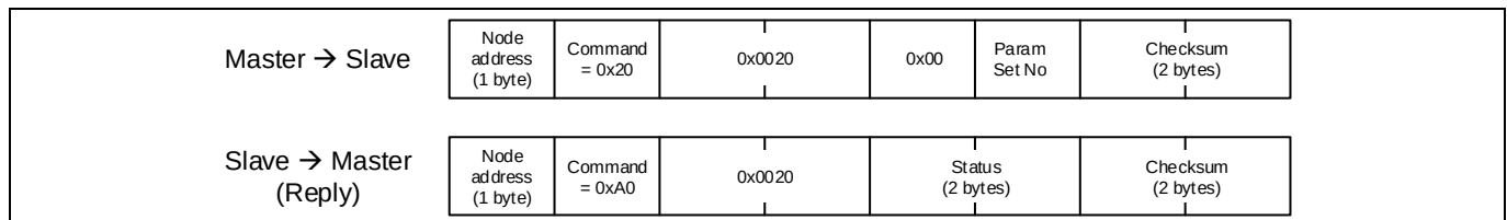
Figure 35 Load parameter Command
