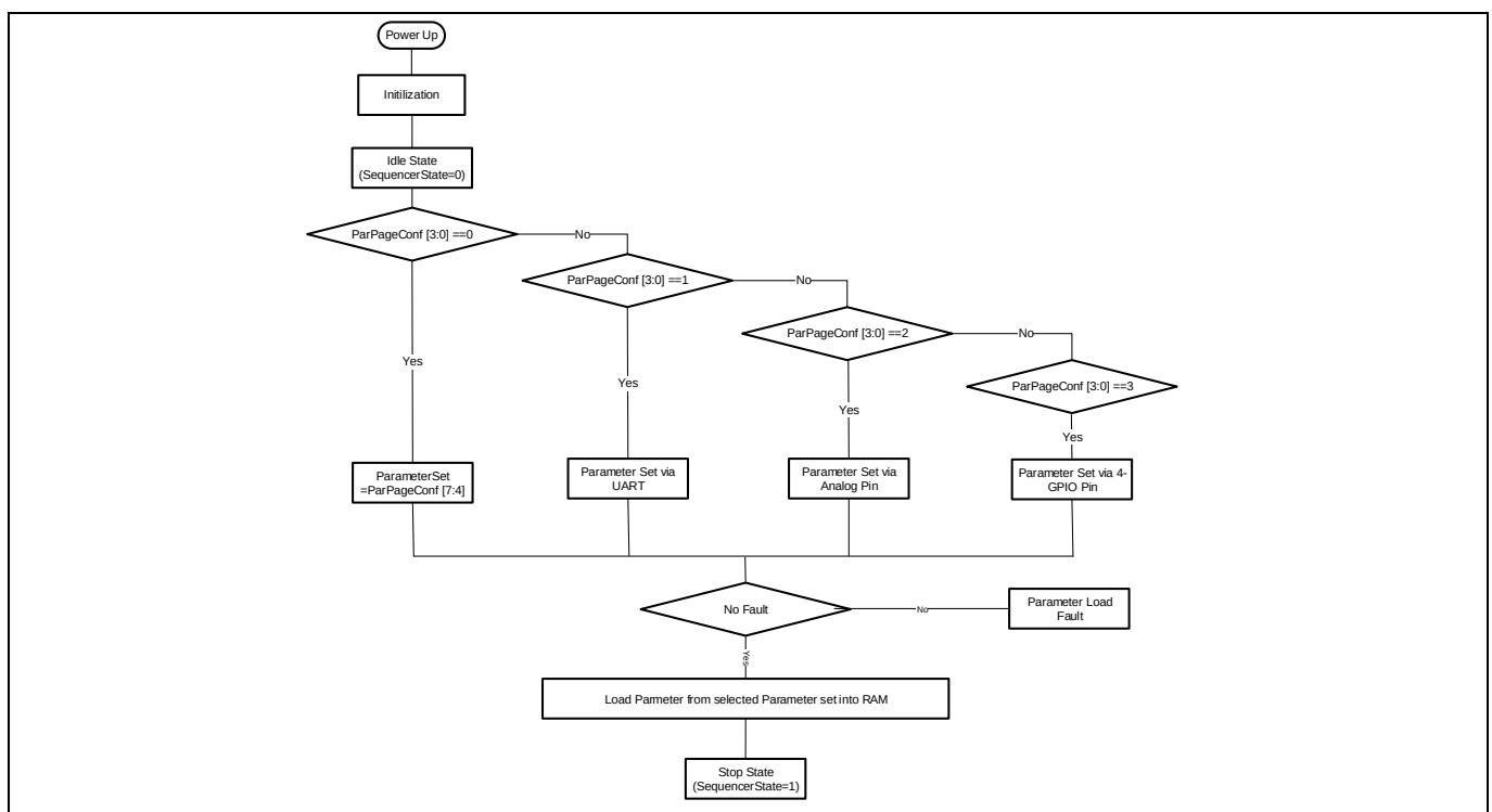
Figure 38 Parameter Load Procedure
