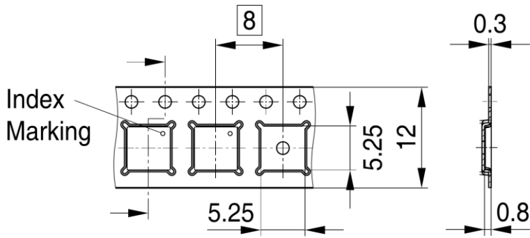
LG-UIQFN-32-2, -3-TP V02
