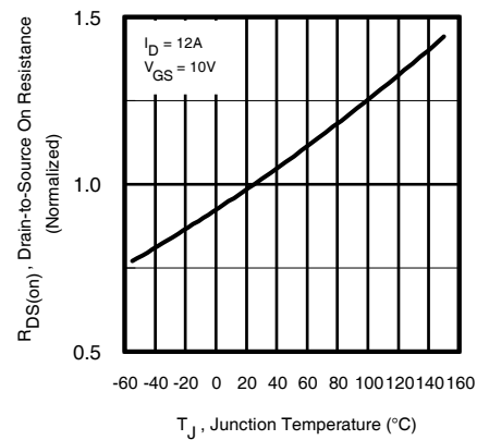
Q2 - Synchronous FET
