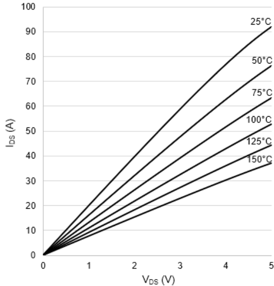
I_{DS} vs. V_{DS} , T_J dependence
