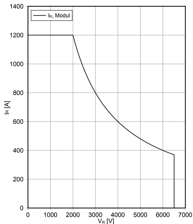
安全動作領域 Diode、インバータ (SOA) safe operation area Diode, Inverter (SOA)
