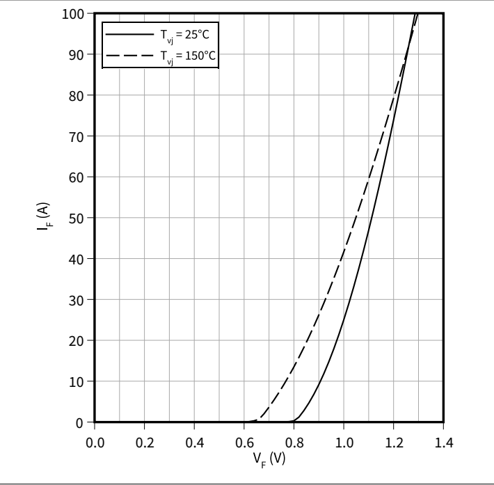
正向特性（典型), 二极管, 整流器
