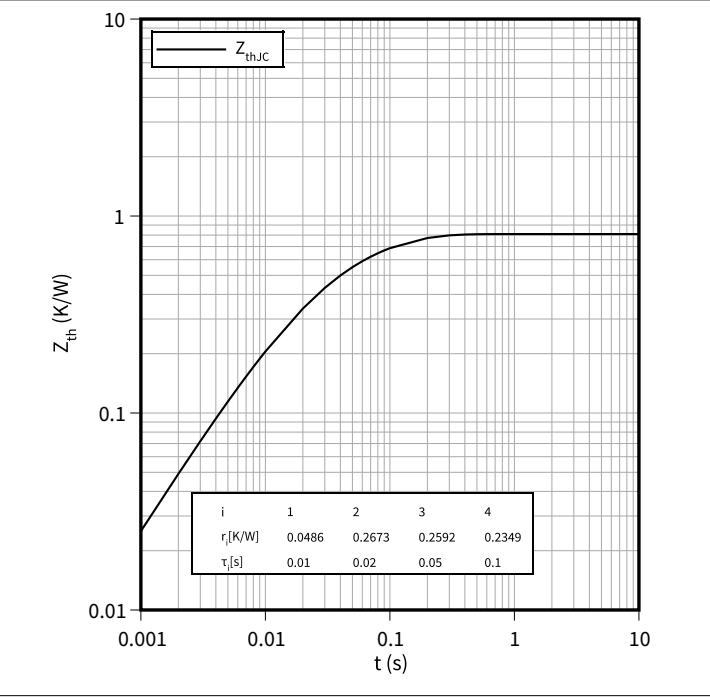
瞬态热阻抗, 二极管, 逆变器
