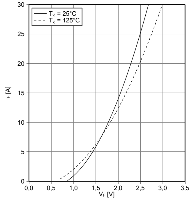
順電圧特性 Diode、ブレーキチョッパー ( typical) forward characteristic of Diode, Brake-Chopper (typical) I_F = f(V_F)
