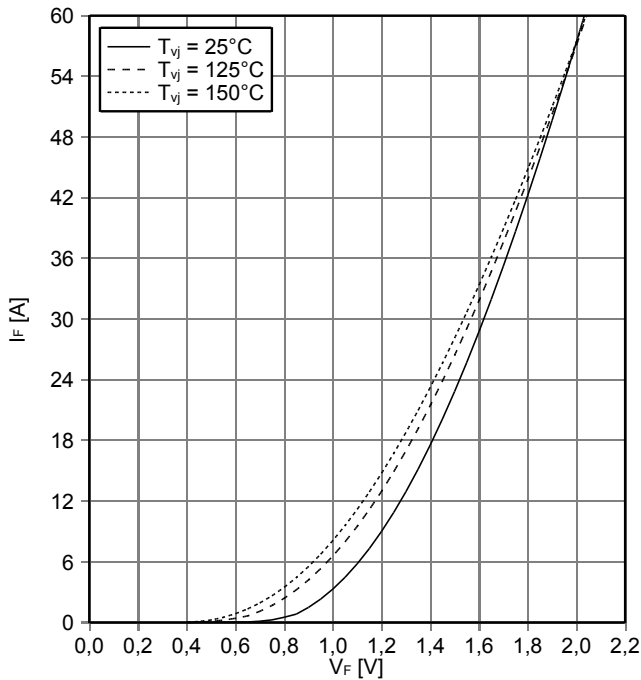
順電圧特性 Diode、ブレーキチョッパー ( typical) forward characteristic of Diode, Brake-Chopper (typical) I_F = f(V_F)
