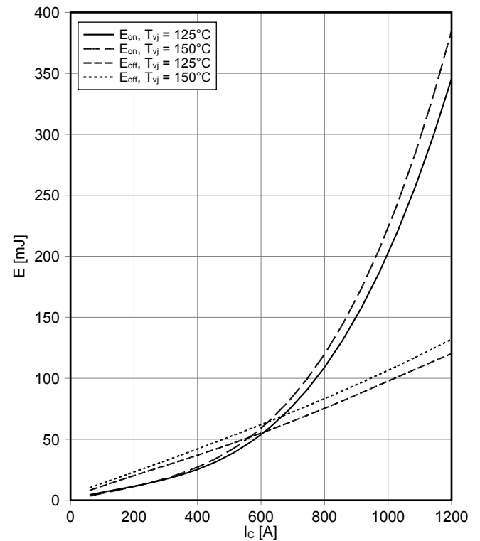
スイッチング損失 IGBT- インバータ (Typical) switching losses IGBT, Inverter (typical) E_{on} = f(I_C) , E_{off} = f(I_C) V_{GE} = \pm 15\text{ V} , R_{Gon} = 1.3\ \Omega , R_{Goff} = 1.3\ \Omega , V_{CE} = 400\text{ V}
