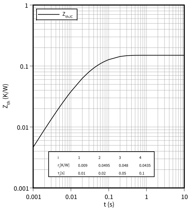
瞬态热阻抗, 二极管, 逆变器
