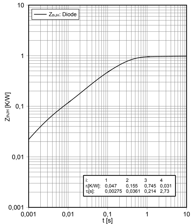
過渡熱インピーダンス Diode、整流器 transient thermal impedance Diode, Rectifier Z_{thJH} = f(t)
