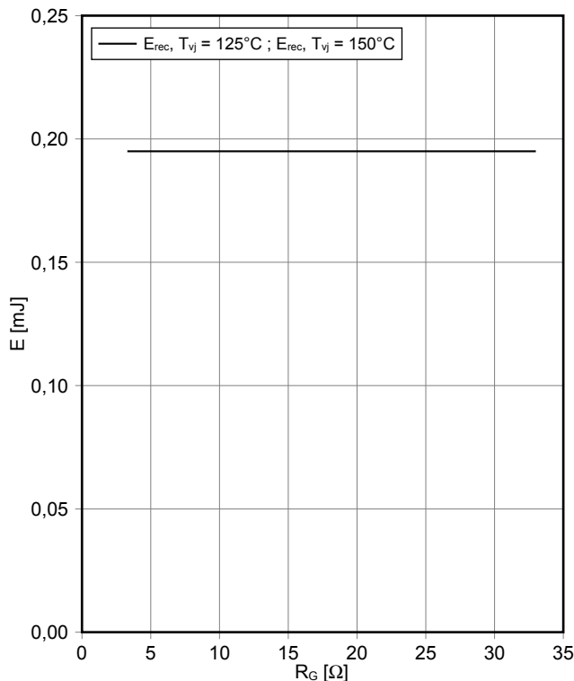
スイッチング損失 ダイオード、スリー・レベル (Typical) switching losses Diode, 3-Level (typical) E_{rec} = f(R_G) I_F = 60 A, V_{CE} = 600 V
