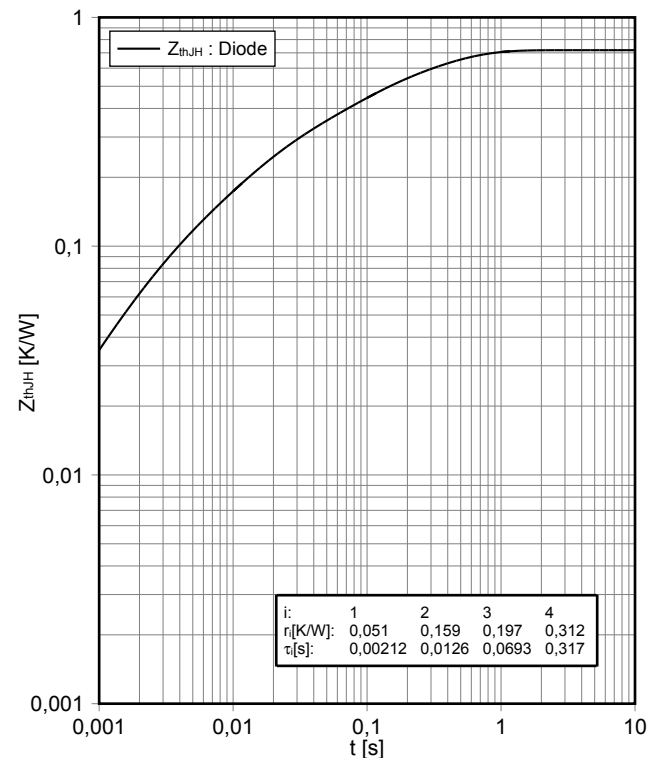
過渡熱インピーダンス ダイオード、スリー・レベル transient thermal impedance Diode, 3-Level Z_{thJH} = f(t)
