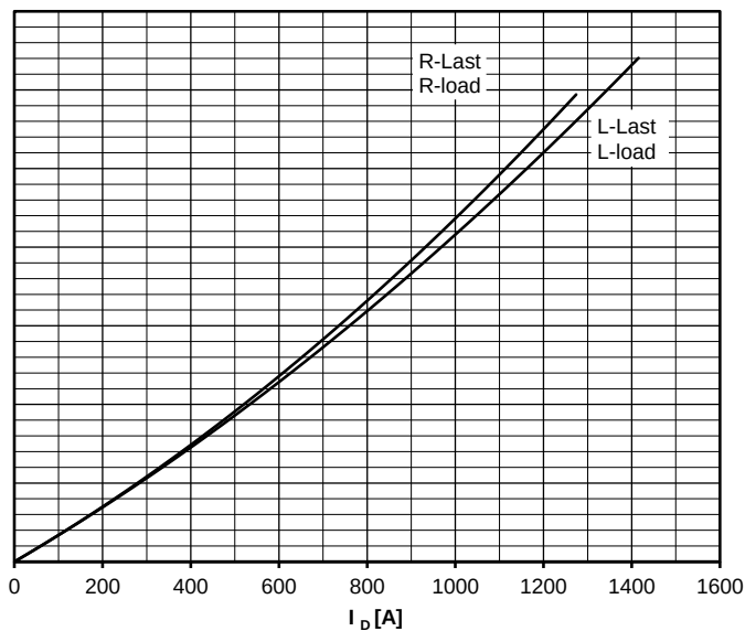
Höchstzulässiger Ausgangsstrom / Maximum rated output current I_D
